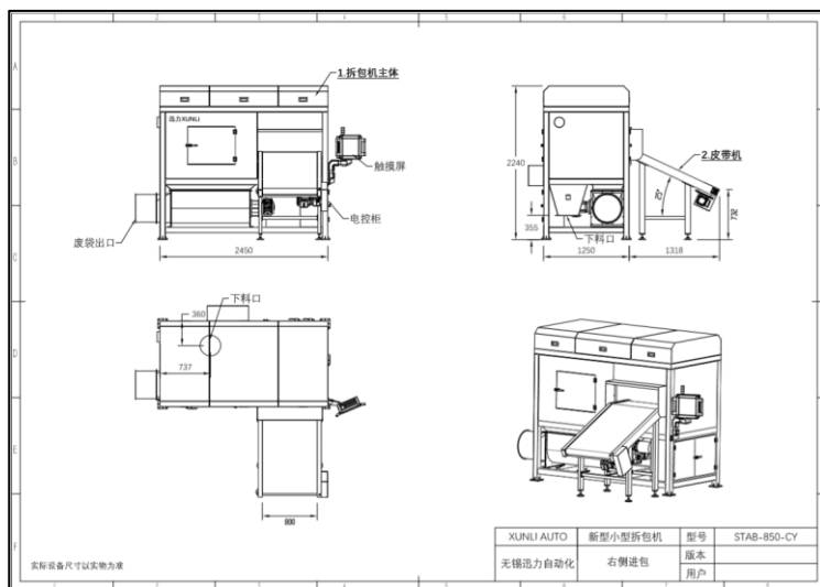
STAB-850 小型自动拆包机标准版三视图
